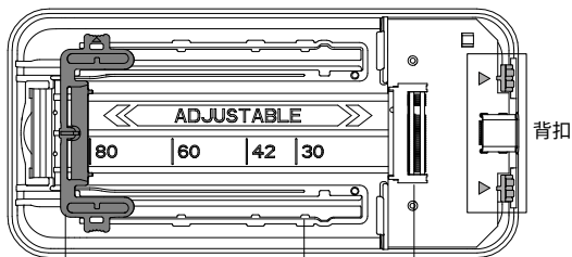
可调M.2 SSD固定器
